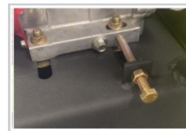
Perno de fácil acceso para tensar faja ahorra tiempo de ajuste
